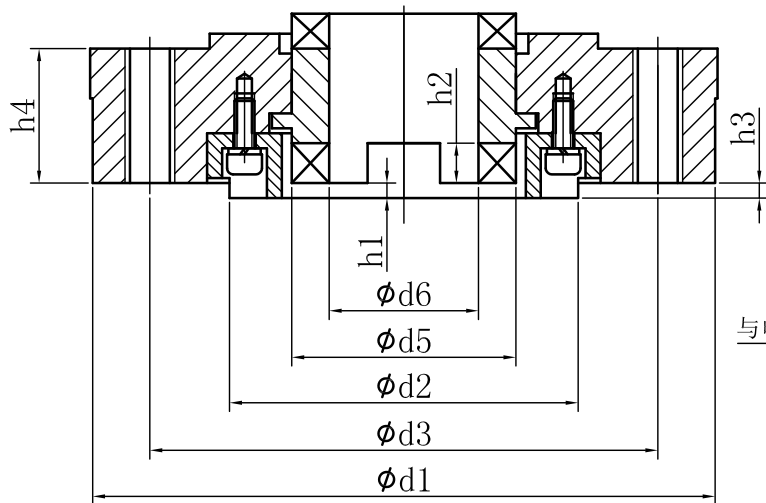
IMC系列GB/T12222 (ISO5210) 法兰型式连接尺寸
